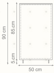
ELEVACIÓN LATERAL
