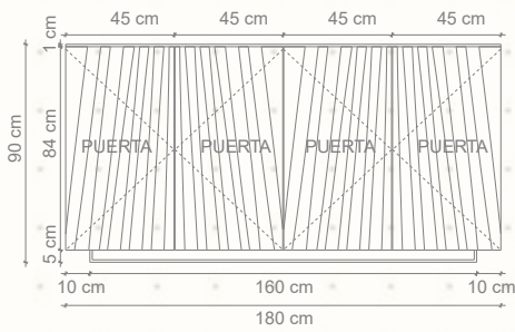
ELEVACIÓN FRONTAL
