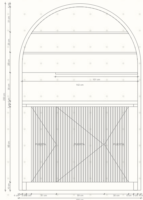
ELEVACIÓN FRONTAL
